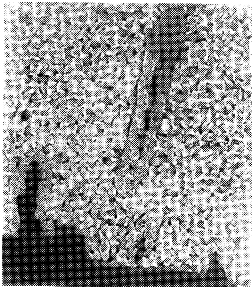
а, б — внешний вид; а — микроструктура 100 X; з — микроструктура в зоне дефекта 300
